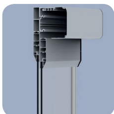
Detalle sección vertical superior
