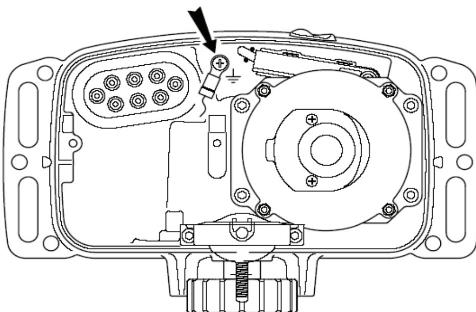
Conexiones para la toma de tierra
