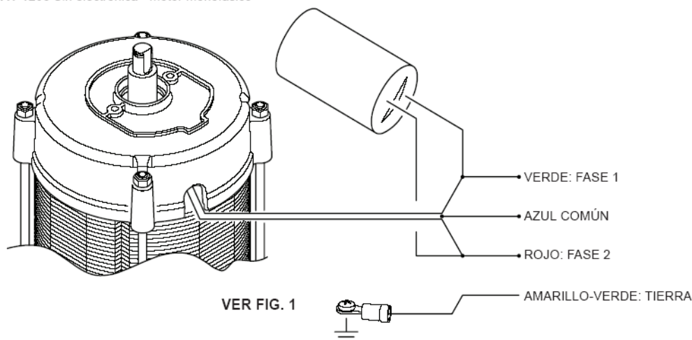
AT 120e Sin electrónica - motor monofásico
